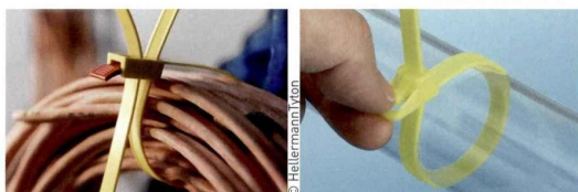
Ce collier de 760 mm de long est facile à ouvrir à l'aide de son levier rouge. Le collier ORF demeure le plus rapide à mettre en œuvre et à ouvrir.
